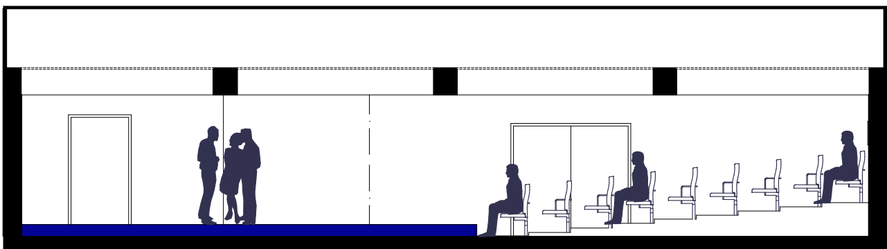
PREREZ C-C
