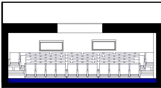
PREREZ B-B
